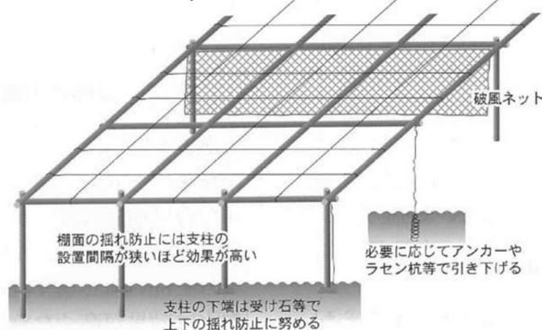
図1 パイプの補強、破風ネット
