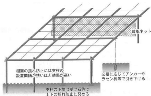
図1 パイプの補強、破風ネット
