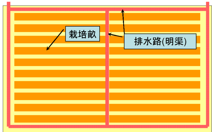
【赤線部分に排水路（明渠）を設置した例】 （ほ場長辺を分断するように明渠を設置）
