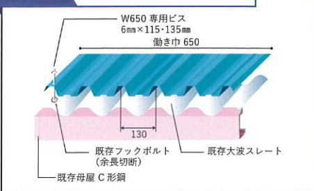
構成図 スレート大波 SS-W650
