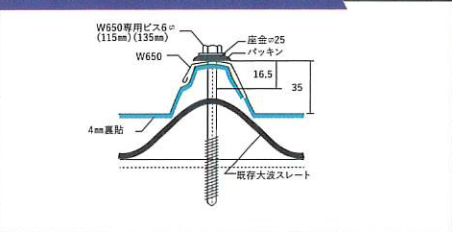
大波スレート屋根改修工法図
